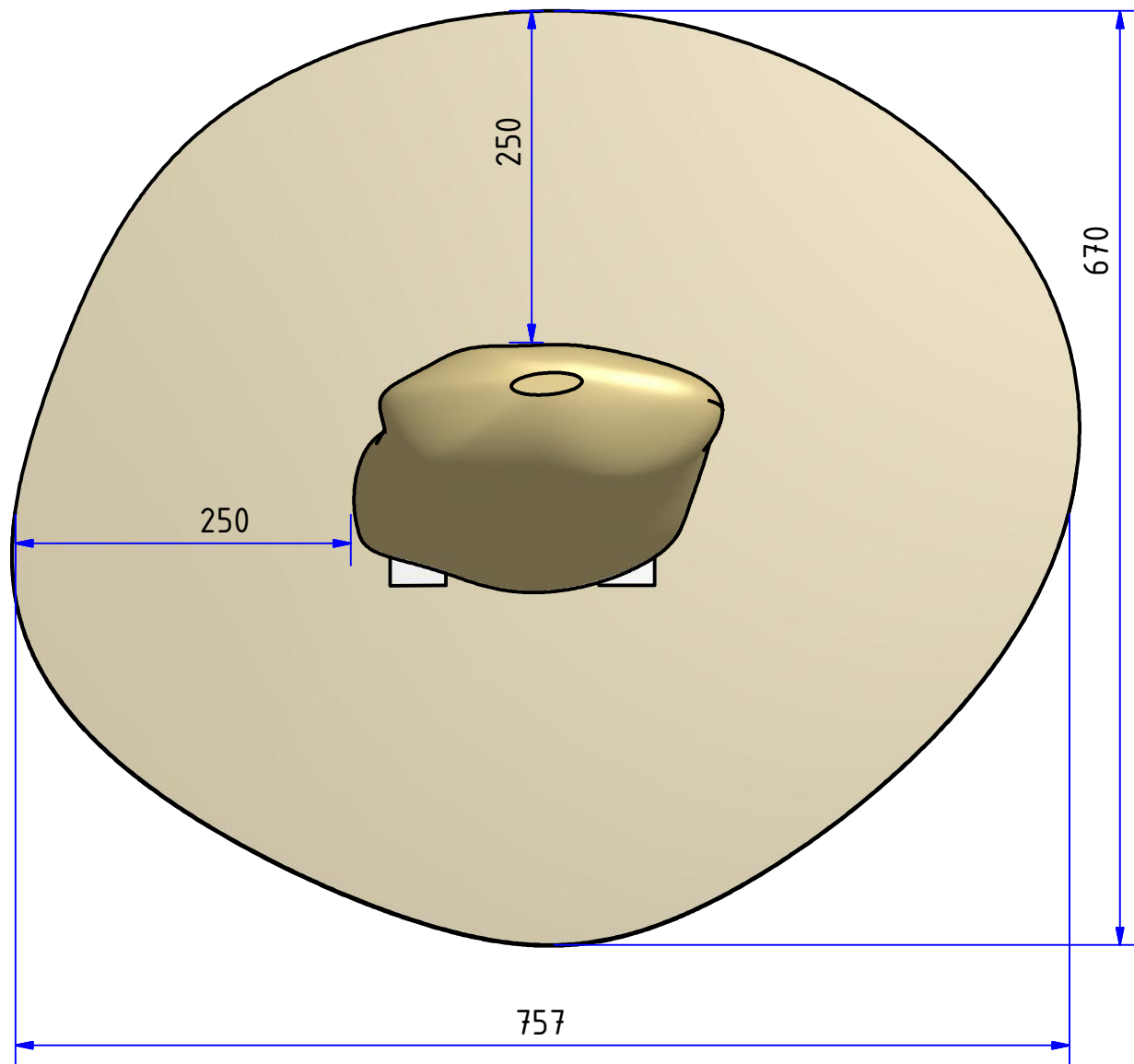
Půdorys dopadiště
